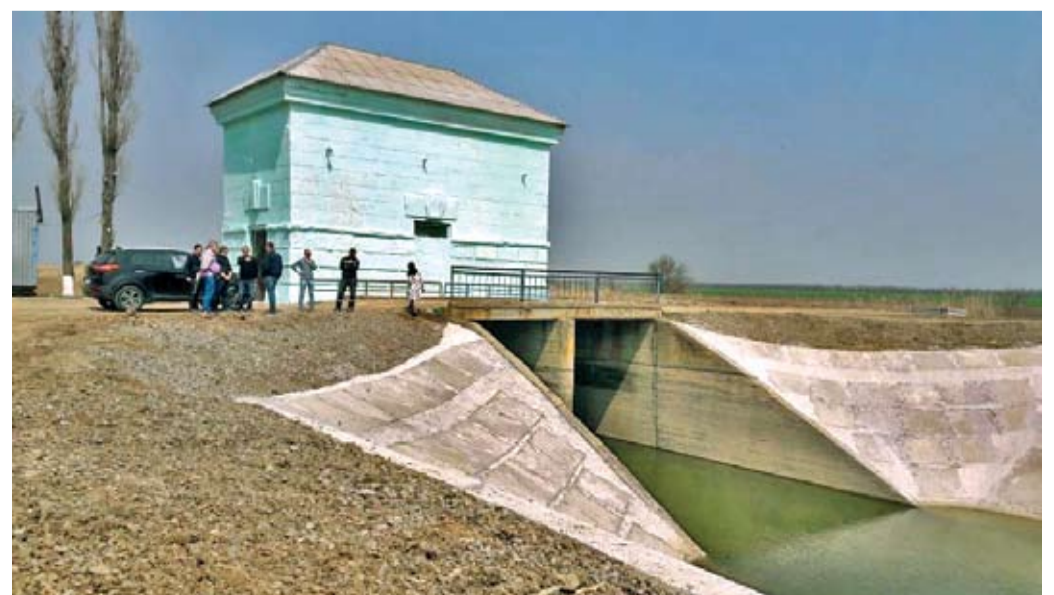
Отремонтированное ГТС
